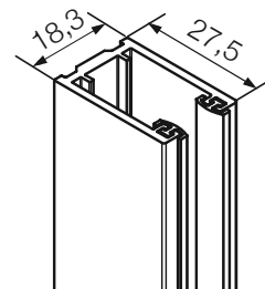
Guida autoportante FD cod. 945
