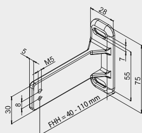
Squadretta per guide in ghisa tipo 2
