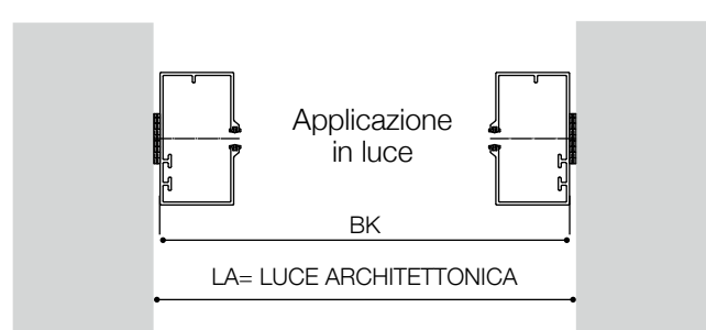
Guida con aletta - cod. 964
