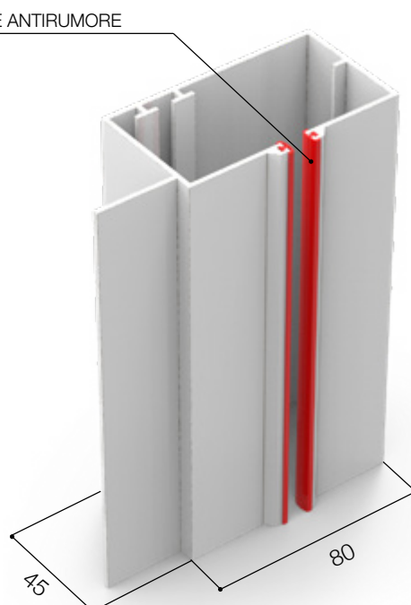
Guida con aletta - cod. 964
