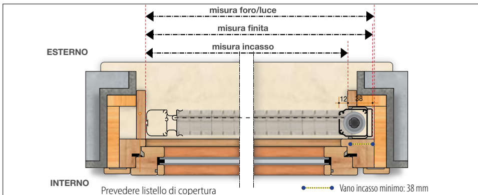
Sezione orizzontale con opzione "Incasso 2 lati".
