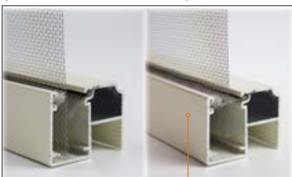
Guida con sistema antivento (brevetto internazionale Bettio)
