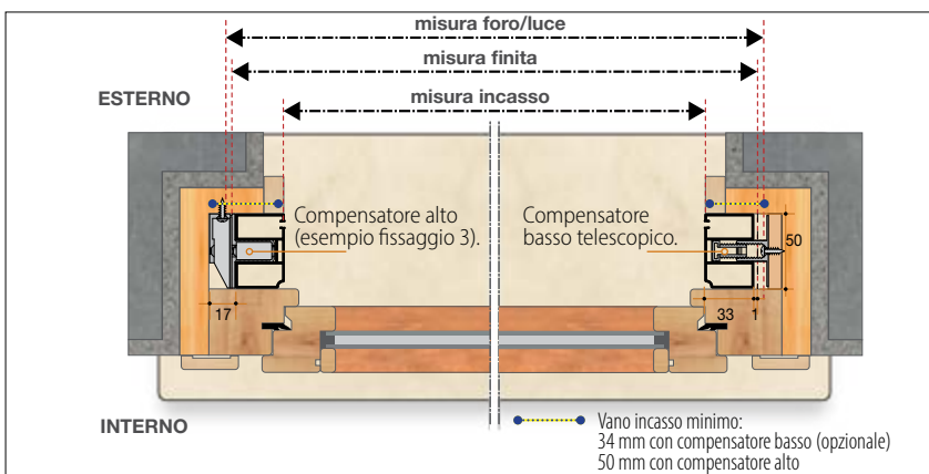
Sezione orizzontale
